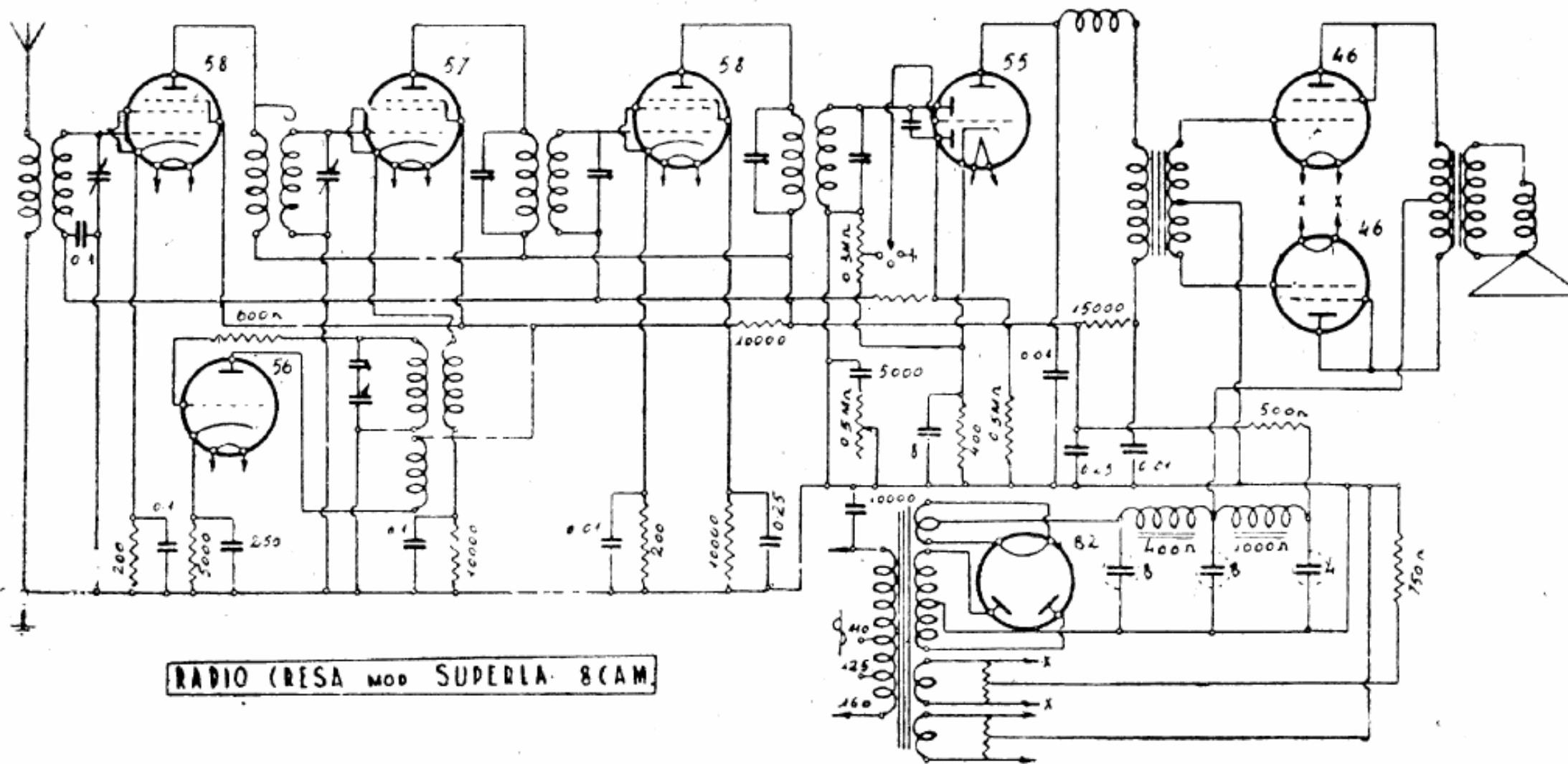
RADIO CRESA — Modelli: « Superla 8 CAM » e « Superla 80 » - Produzione 1934 Media frequenza: 175 kc
